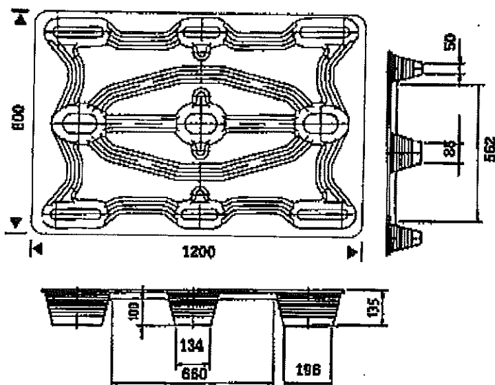
Esquema F 8 LF Euro-Palet 800 x 1200 mm
